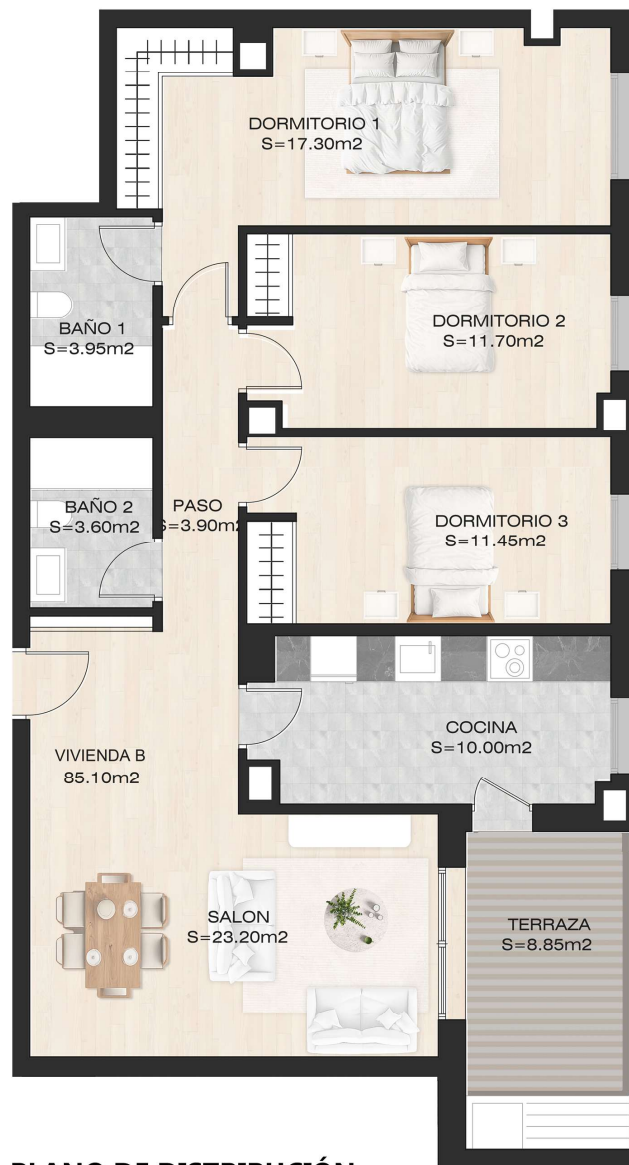
PLANO DE DISTRIBUCIÓN VIVIENDA B - PLANTA 1-4
